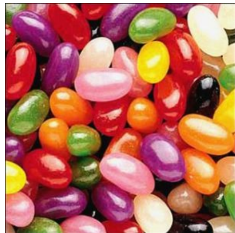
jellybeans
