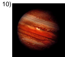
Jupiter
